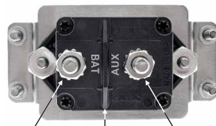
Battery 1/4"-28 Input Stud Stud Barrier Auxiliary 1/4"-28 Output Stud
